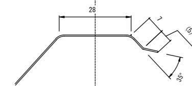
B 部下重ね詳細 (1:1)
