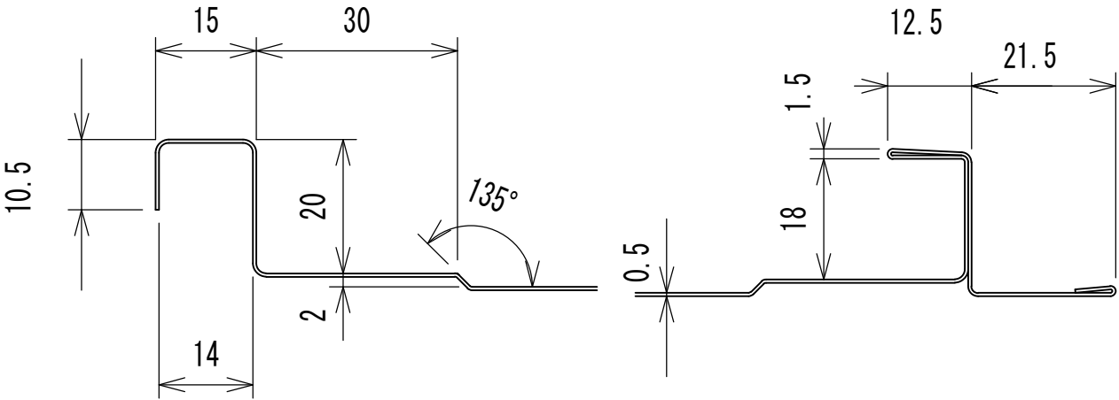
寸法詳細図
