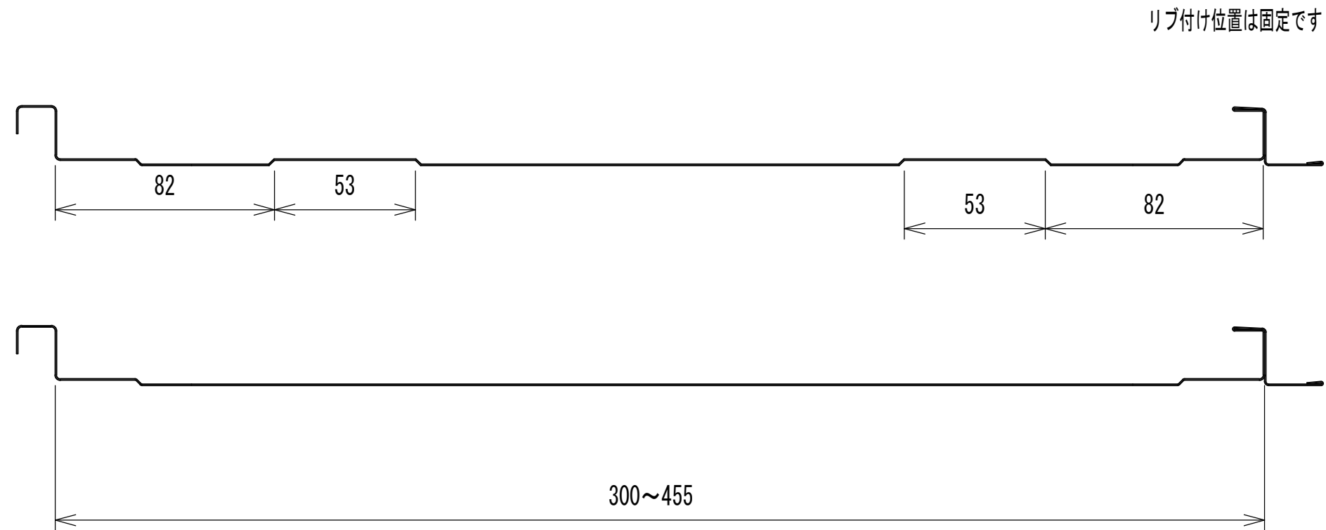
製品図
