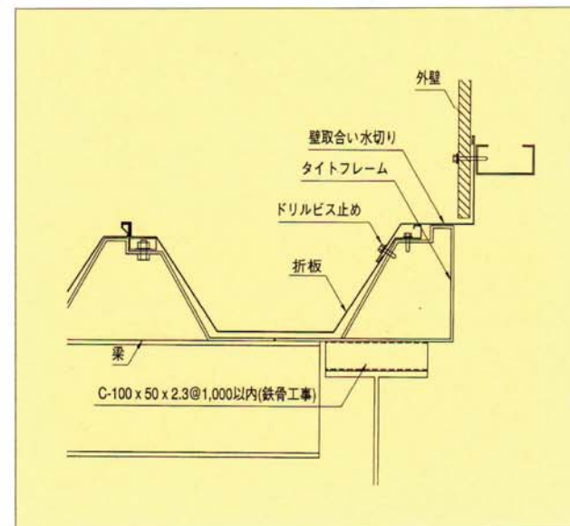
■壁取合い納め図
